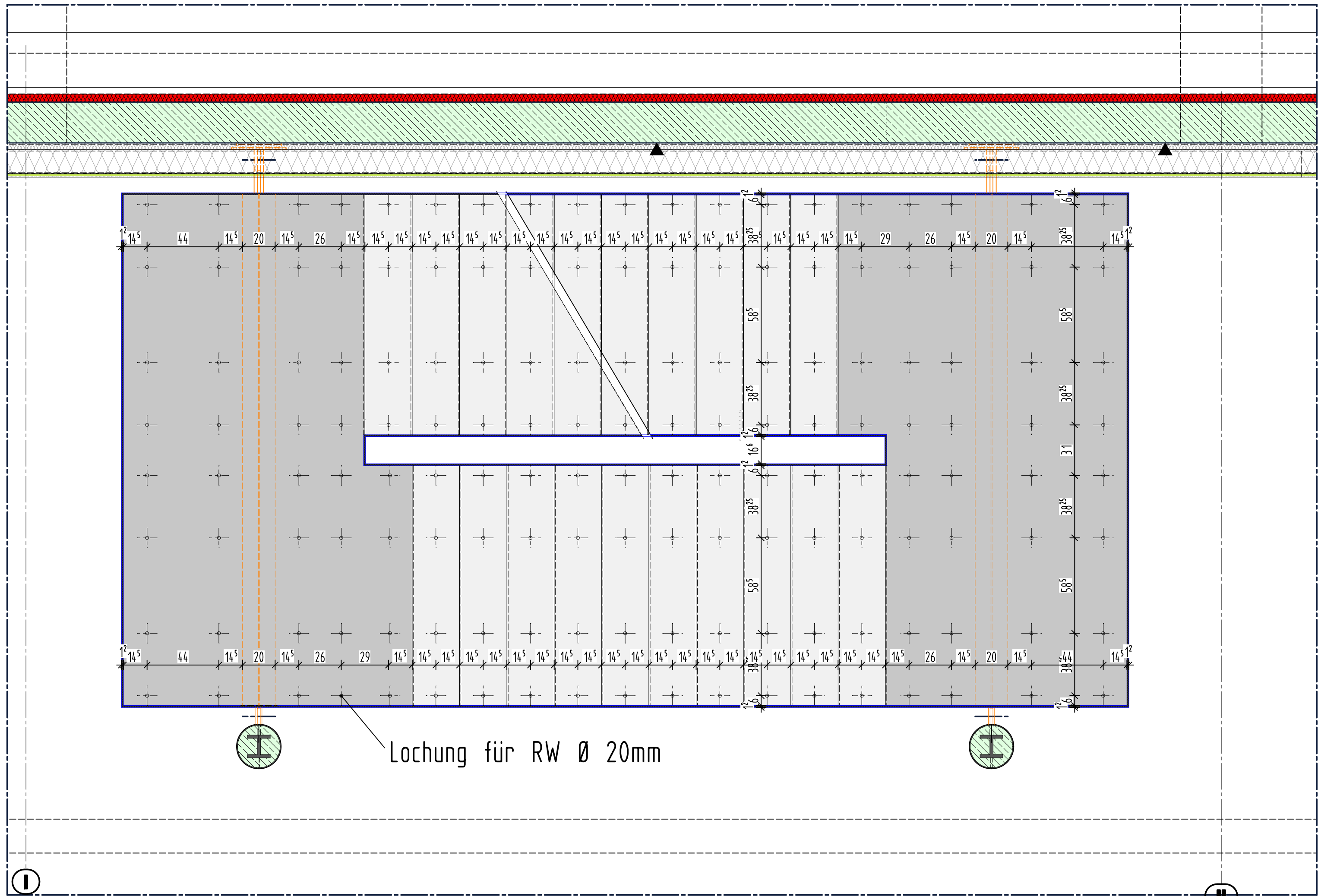
Übersicht Lochung für RW M 1:20
