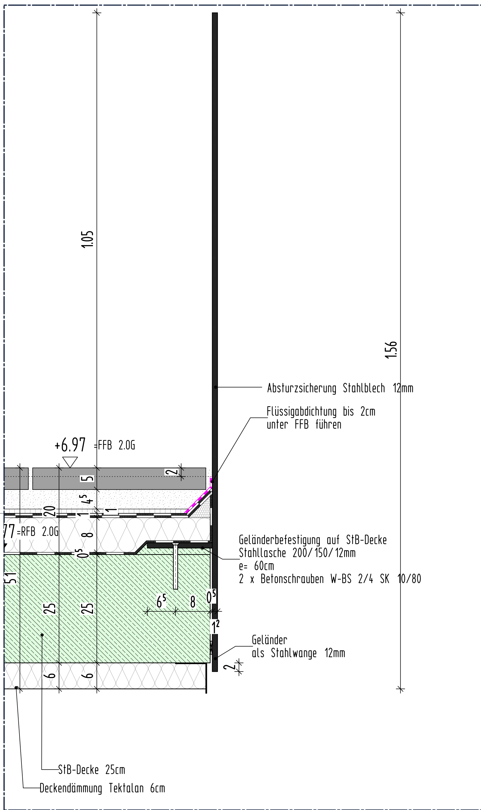
Detailschnitt DD-DD Geländer Hauptpodest 2.OG M 1:5
