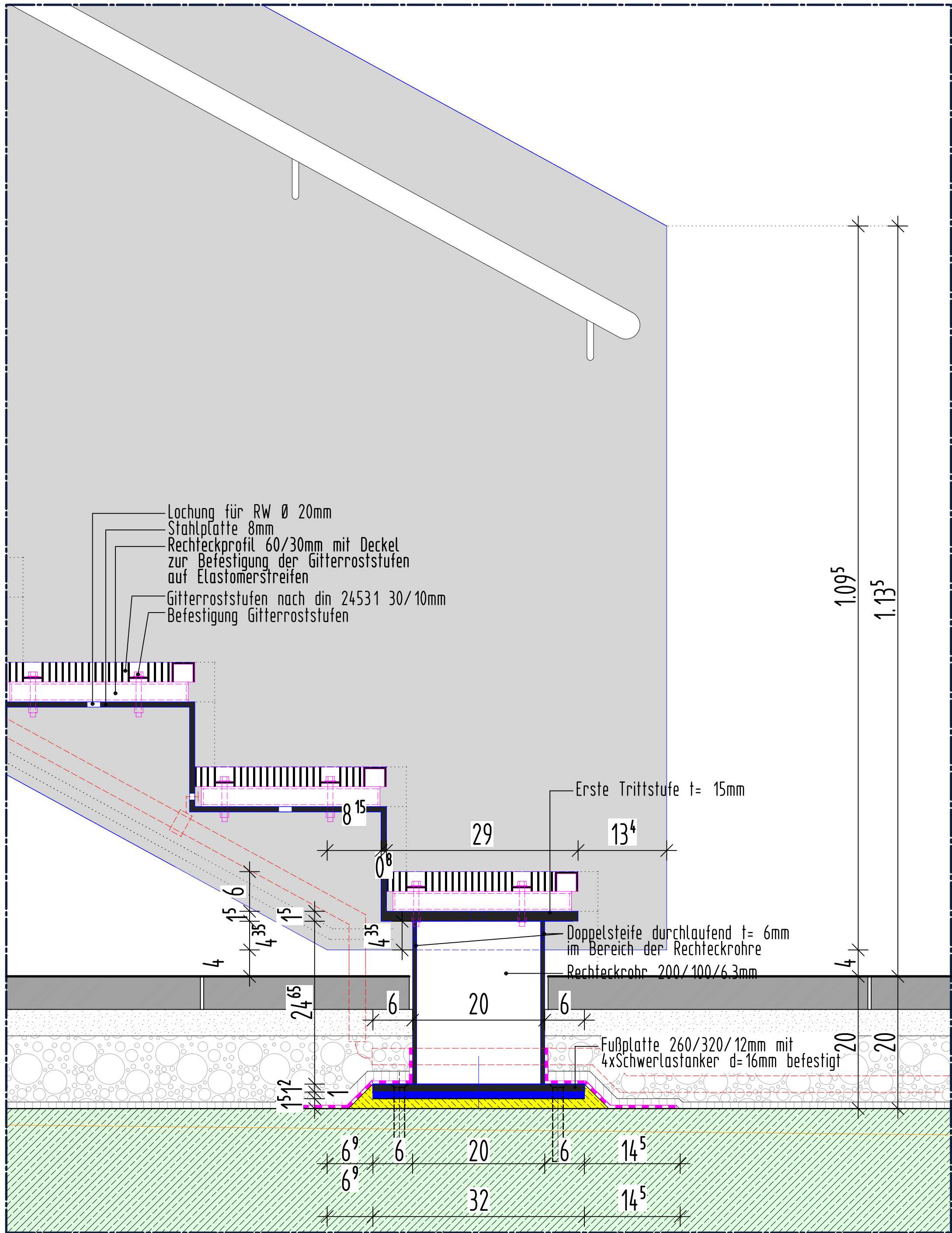
SCHNITT 11-11 Fußpunkt M 1:5
