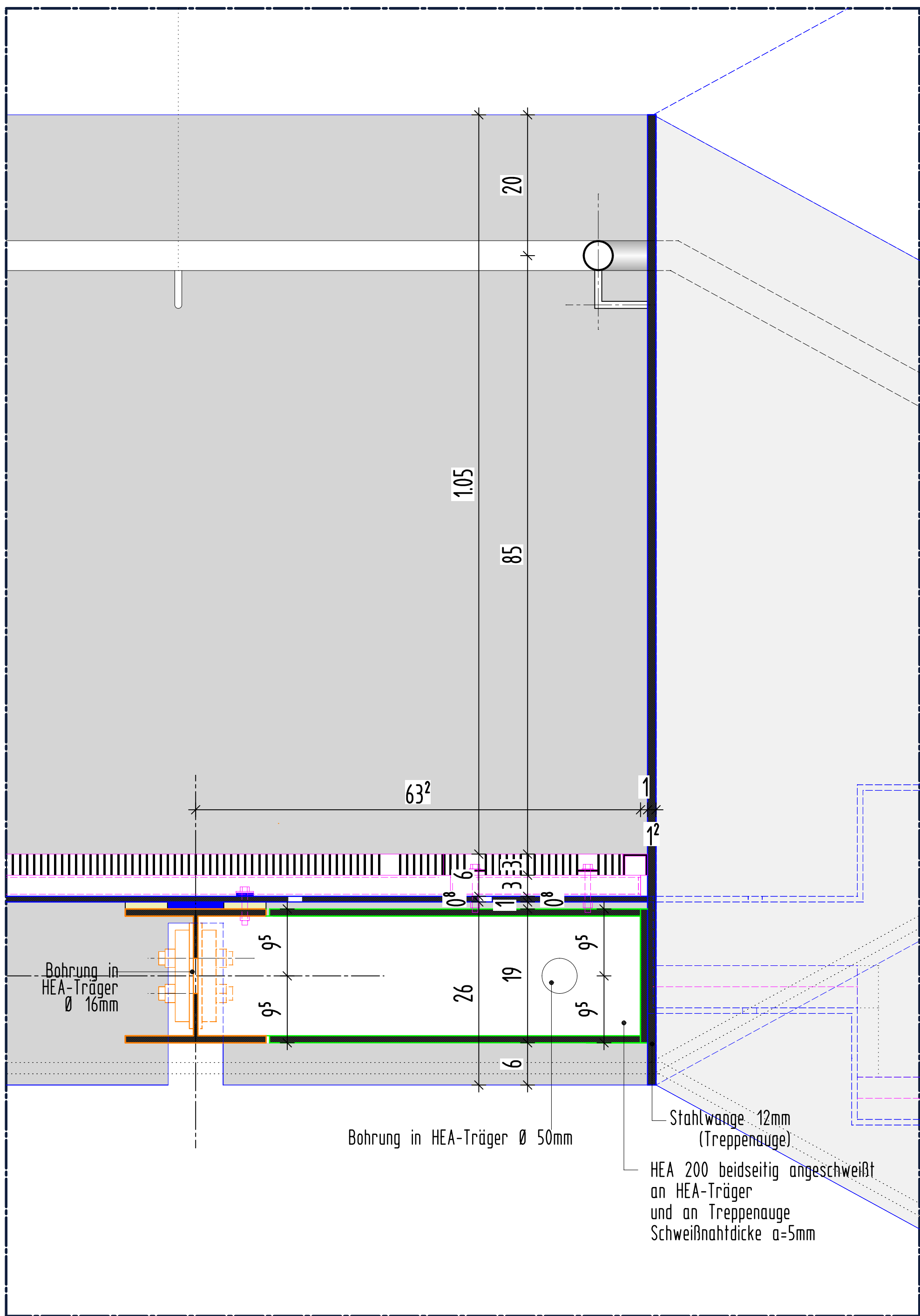
Detail 14-14 durch Treppenaue M 1:5
