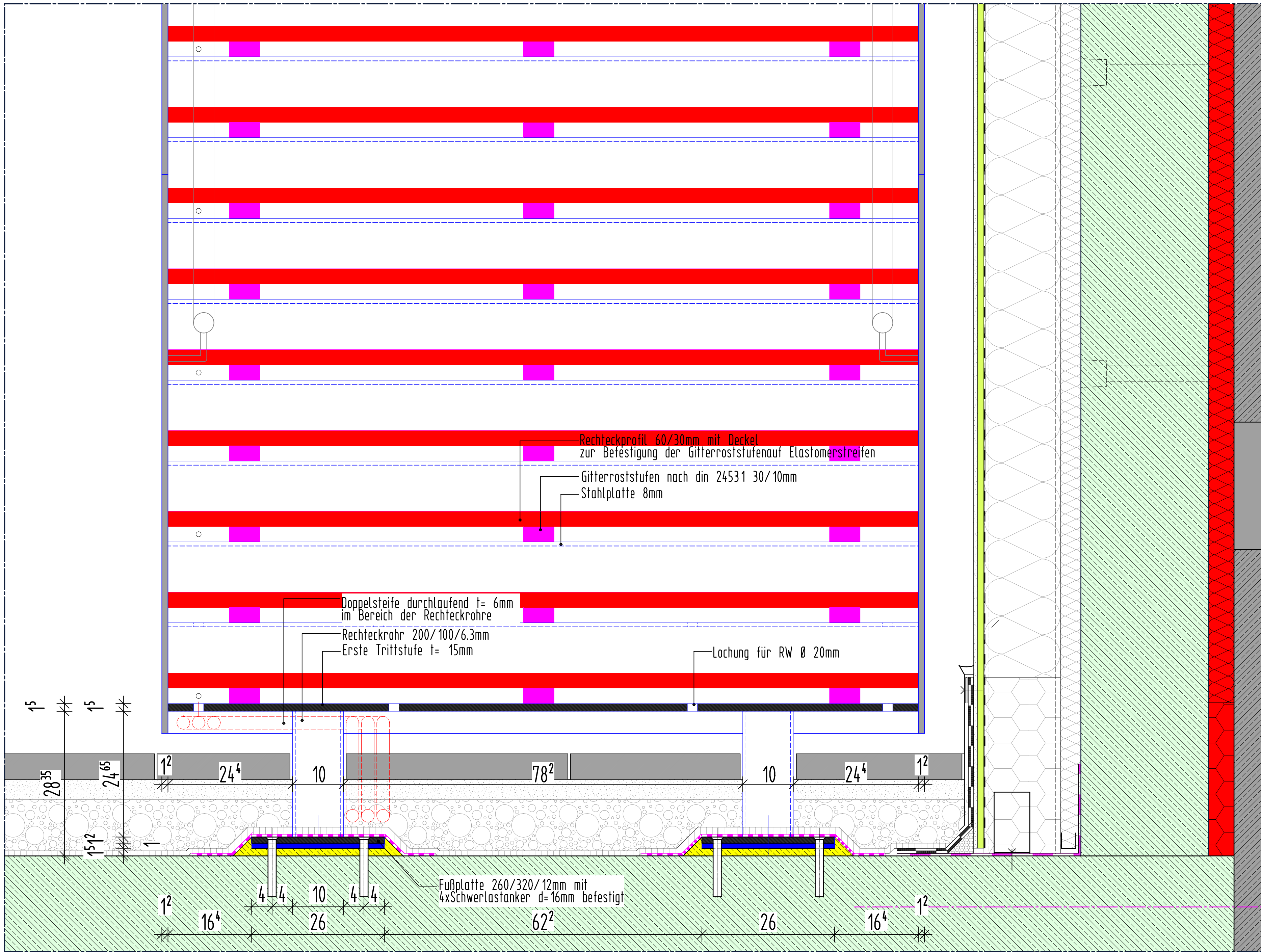
Detail 12-12 Fußpunkt M 1:5
