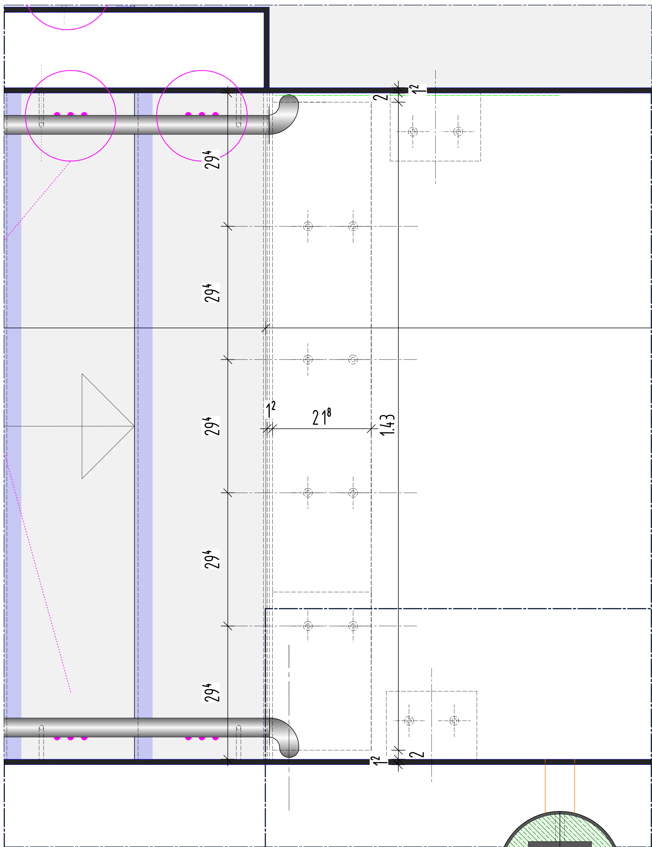
Fußpunkt 13-13 2.OG auf Podest M 1:5
