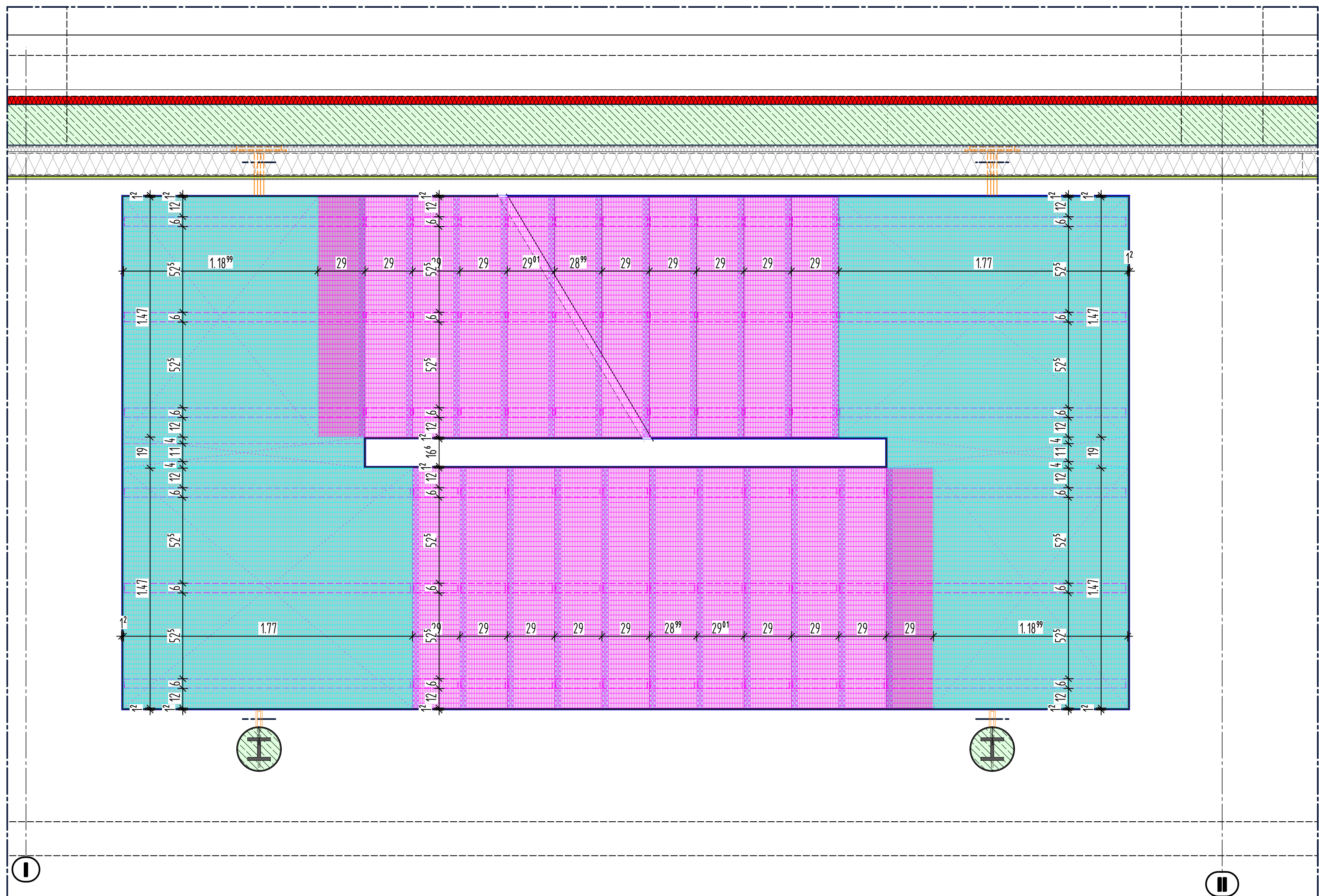
Übersicht Gitterroste M 1:20
